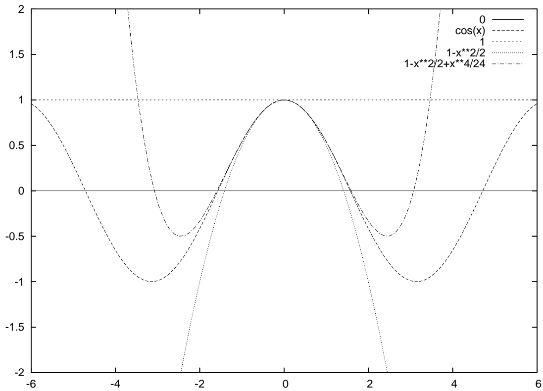
FIG. 3 – cos à l'ordre 4 en 0
