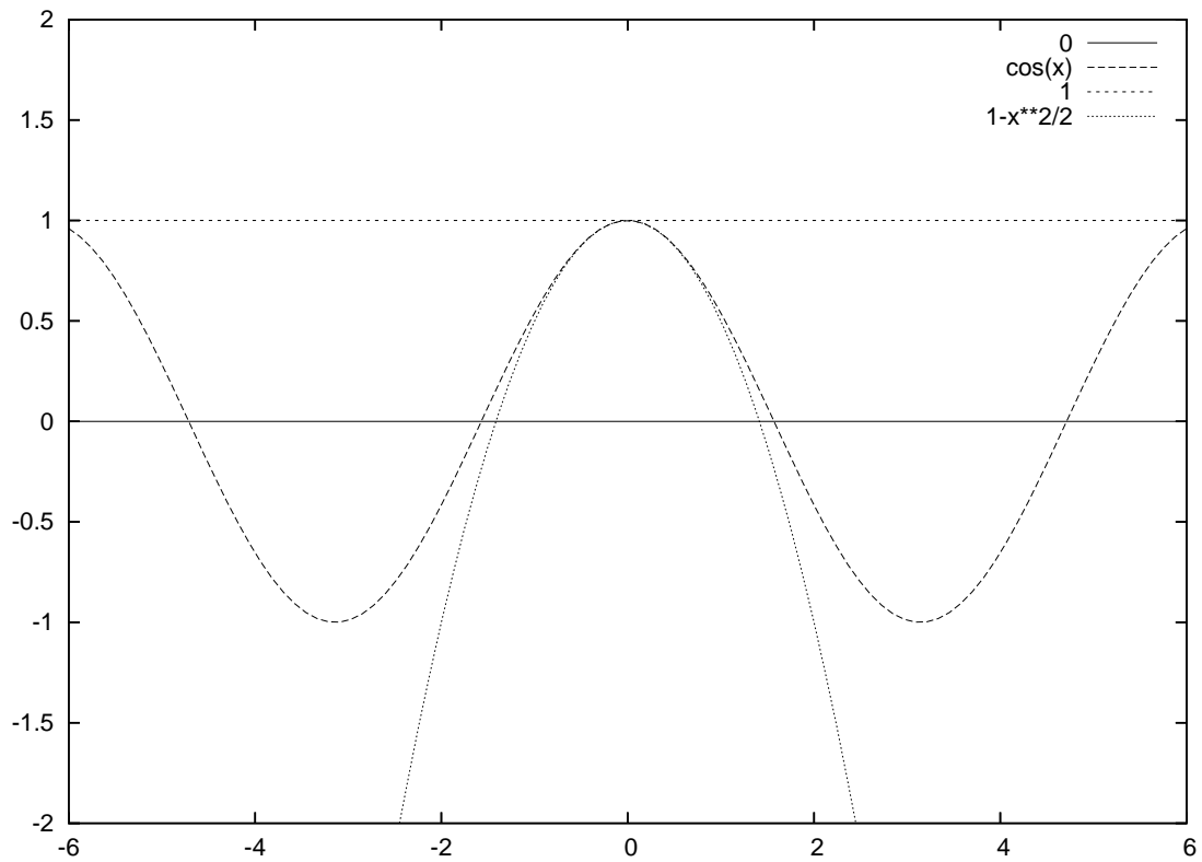
FIG. 2 – cos à l'ordre 1 et 2 en 0
