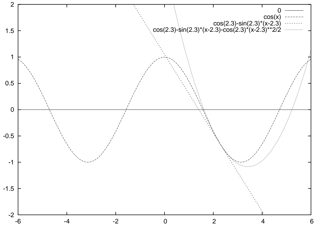
FIG. 1 – cos à l'ordre 1 et 2 en 2,3
