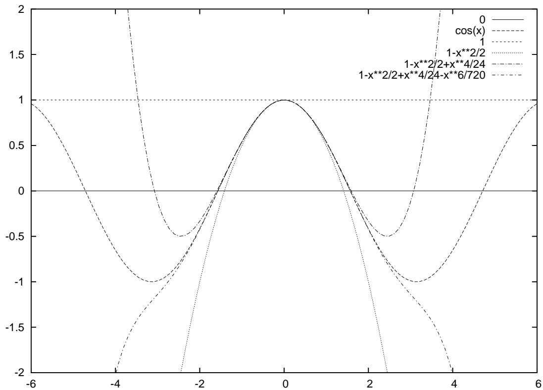
FIG. 4 – cos à l'ordre 6 en 0
